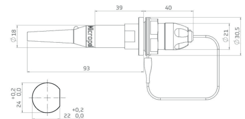
empfohlenes Bohrbild
