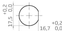
empfohlenes Bohrbild
