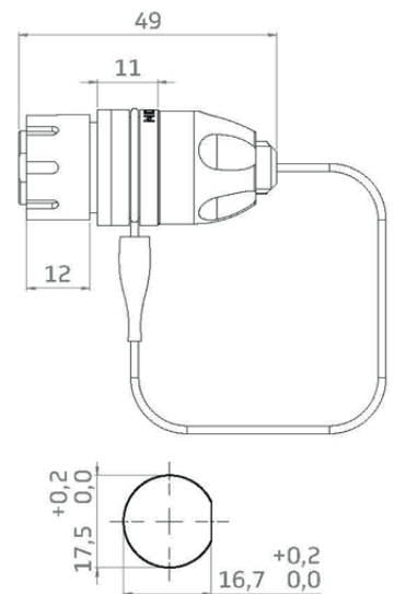
empfohlenes Bohrbild
