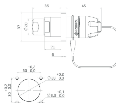
empfohlenes Bohrbild
