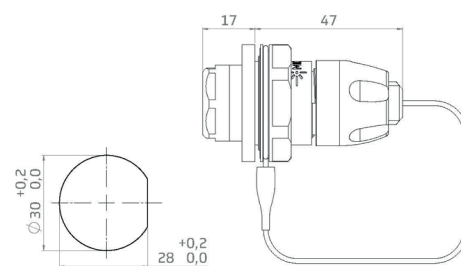
empfohlenes Bohrbild
